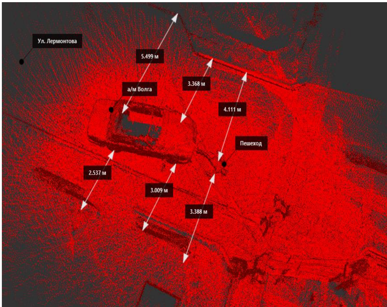
Рисунок 6. 3D-модель наезда а/м «Волга» на пешехода
