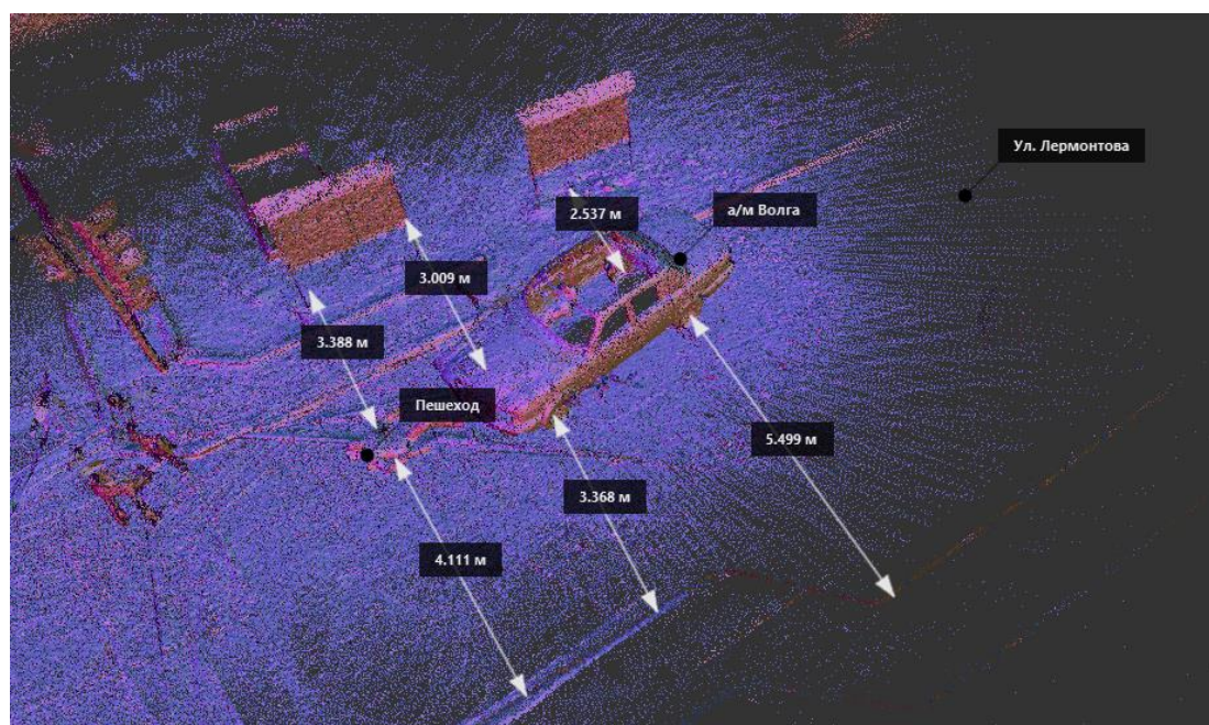
Рисунок 5. 3D-съемка наезда а/м «Волга» на пешехода
