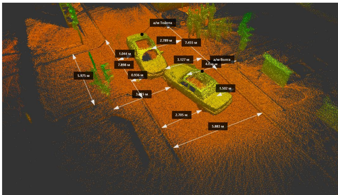
Рисунок 9. 3D-модель столкновения а/м «Волга» с а/м «Тойота» на перекрестке
