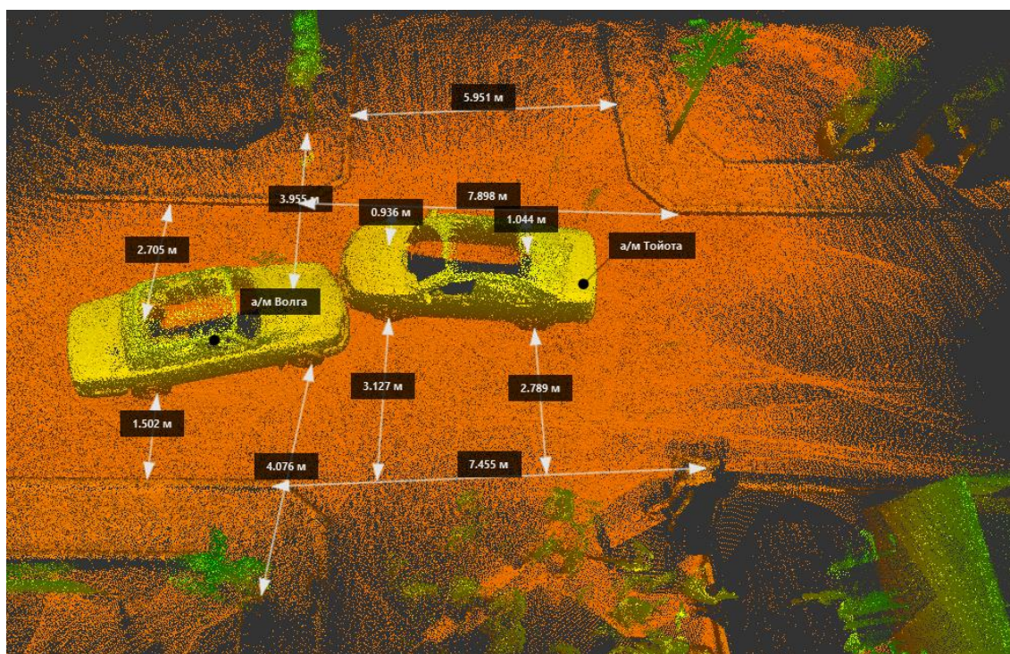
Рисунок 8. 3D-съемка столкновения а/м «Волга» с а/м «Тойота» на перекрестке
